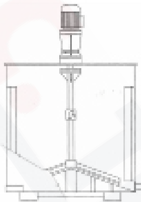
Vasca con fondo conico convesso e agitatore a pale
