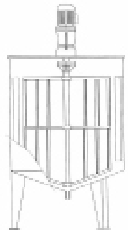
Vasca con fondo conico concavo e agitatore a rastrelliera
